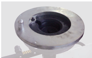
G1000A101 Flangia per autocarri leggeri. Flange for light trucks. LLKW-Flansch. Flasque pour utilitaires. Garra para camiones ligeros/furgonetas.
