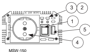
MSW-150
