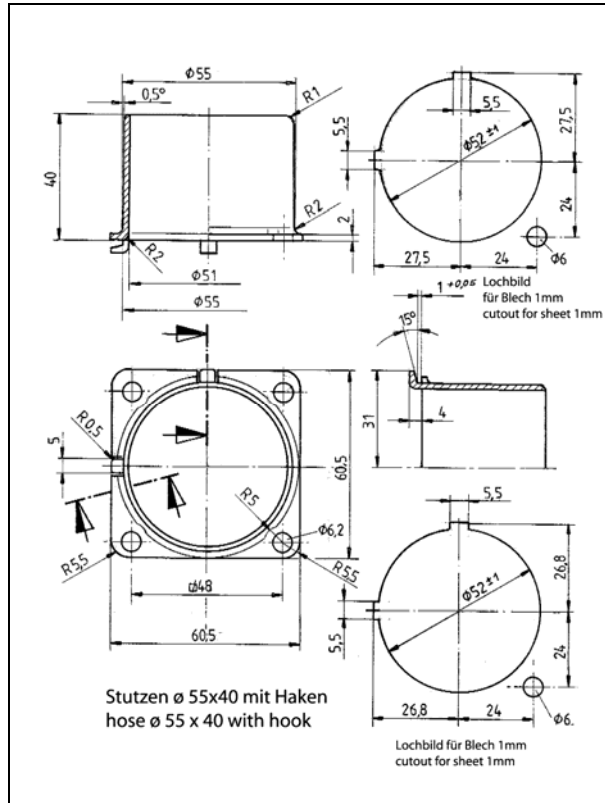
Slangstos Ø 55 mm, höjd 40 mm
