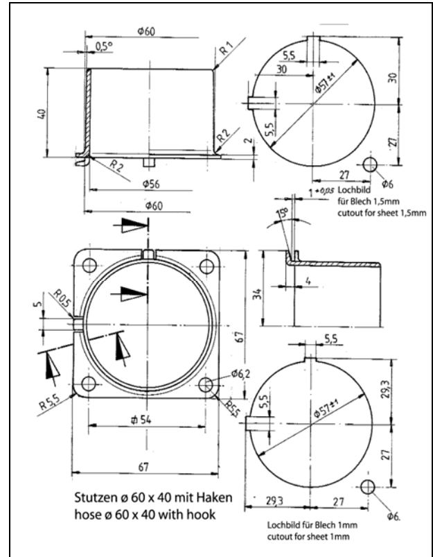
Slangstos Ø 60 mm, höjd 40 mm
