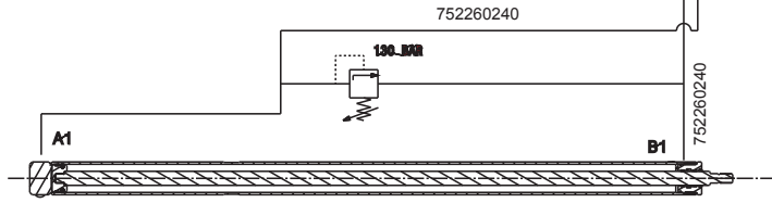
752290530 - CILINDRO TRASLAZIONE CARRO UTENSILE 752290530 - TOOL CARRIAGE TRANSLATION CYLINDER
