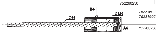
752290780 - CILINDRO APERTURA MANDRINO 752290780 - MANDREL OPENING CYLINDER
