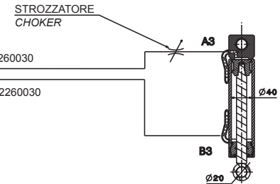
752290242 - CILINDRO ALZATA/BLOCCAGGIO UTENSILE 752290242 - TOOL LOCKING/RAISING CYLINDER
