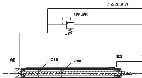
752290410 - CILINDRO TRASLAZIONE CARRO MANDRINO 752290410 - MANDREL CARRIAGE TRANSLATION CYLINDER
