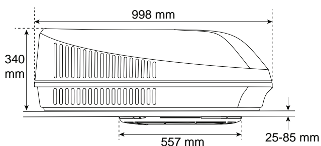
Fig. 03: Monteringsmått (sidovy)
