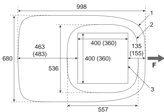
Fig. 02: Monteringsmått vy uppifrån/nerifrån)
