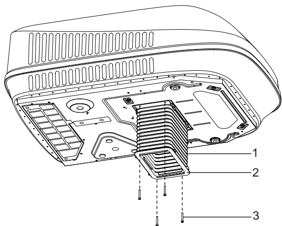
Fig. 12: Installation av luftutloppskanalen
