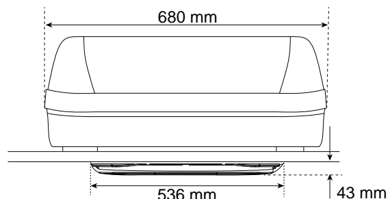
Fig. 04: Monteringsmått (frontvy)
