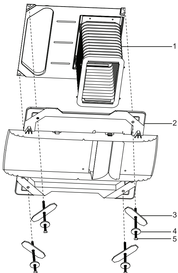
Fig. 14: Montering av M8-bultar
