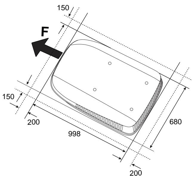
Fig. 01: Monteringsriktning för utomhusenheten
