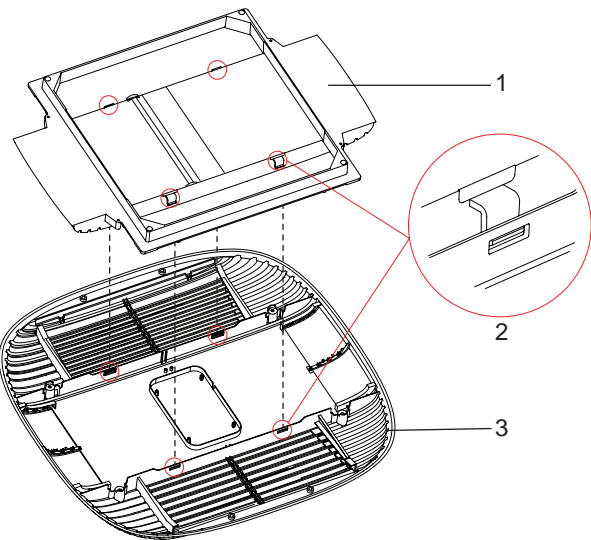
Fig. 18: Fastsättning av luftfördelarenheten på monteringskonsolen
