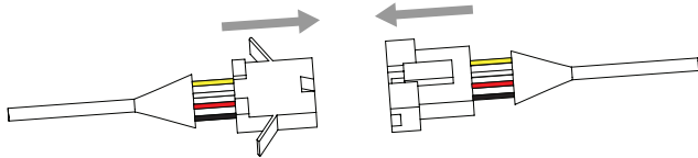
Fig. 17: Anslutning av luftfördelaren - och utomhusenhetens kablar
