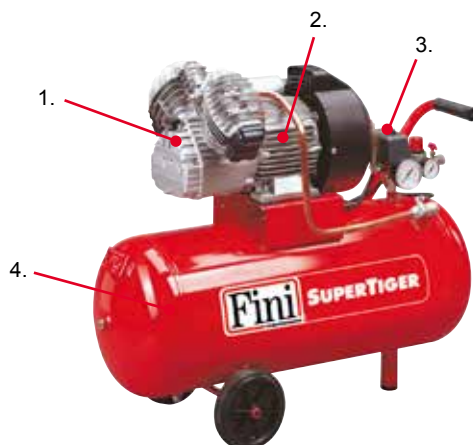
Exempel på direktdriven kolv
