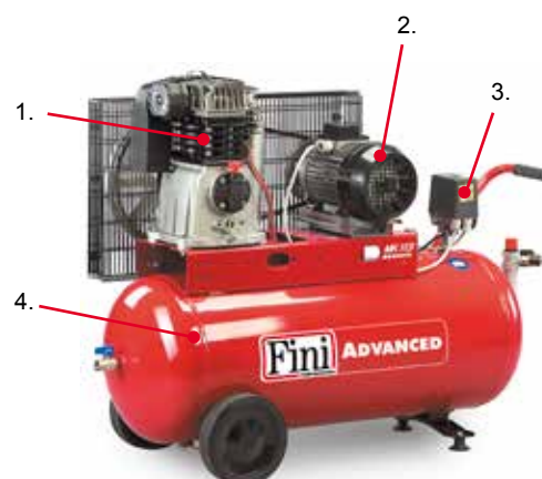
Exempel på remdriven kolv
